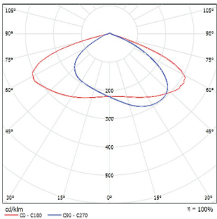
Křivky svítivosti **
